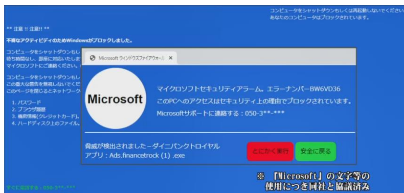
【偽警告画面】
